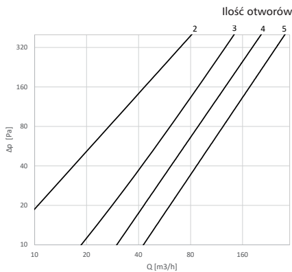
DAT-AKU-125-50 / DAT-AKU-CA-125-50
