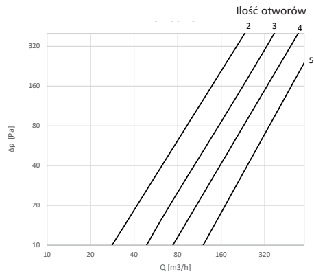
DAT-AKU-200-50 / DAT-AKU-CA-200-50
