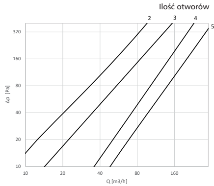
DAT-AKU-100-75
