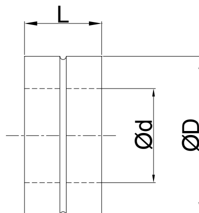
Izolacja 25 mm
